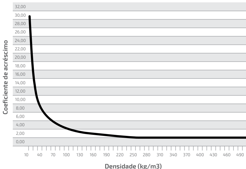
Gráfico 1 - Variação do custo com a densidade da mercadoria (para densidade ideal de 300 kg/m 3 )
